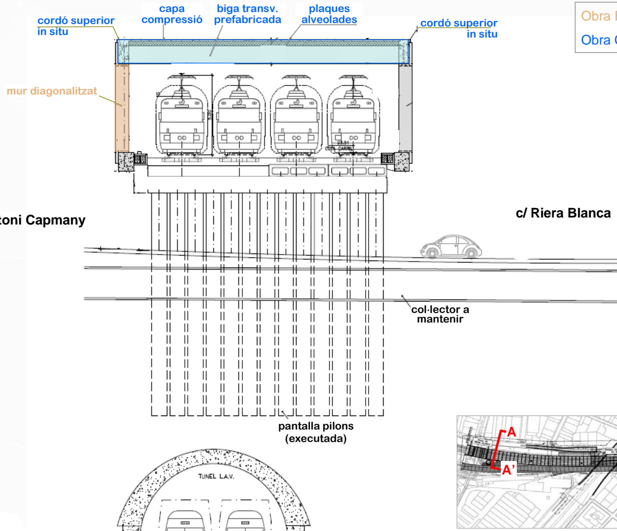
Secció A-A' (pk 1+ 060 eix L.A.V.)
